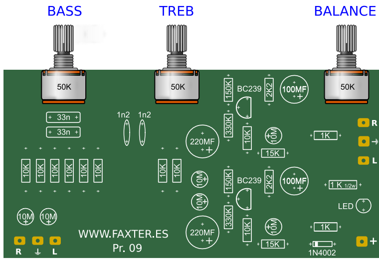
LADO COMPONENTES
